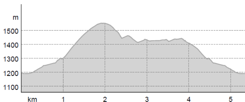
Profilo altimetrico
